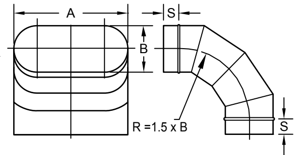
90° ANGLE EASY
