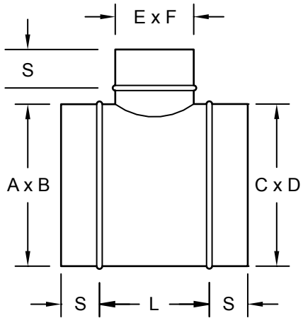
TEE
