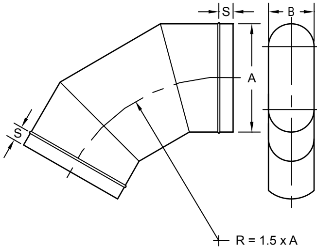
60° ANGLE HARD
